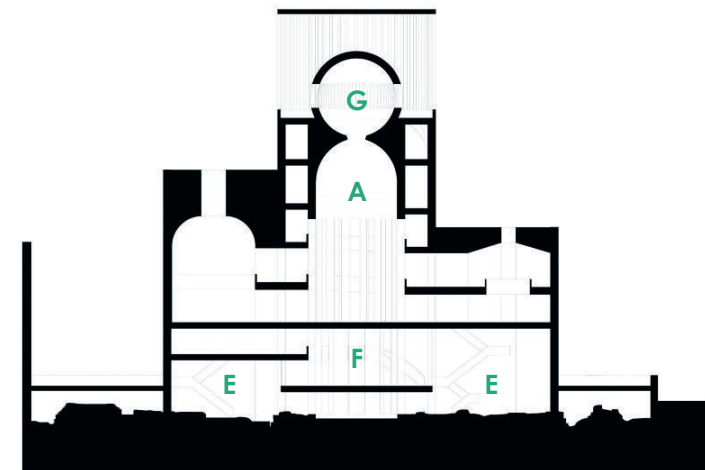
Ábrák: alaprajz és keresztmetszet © Kuehn és Malvezzi
